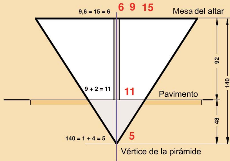
Diseño del altar de la “nueva iglesia”.
