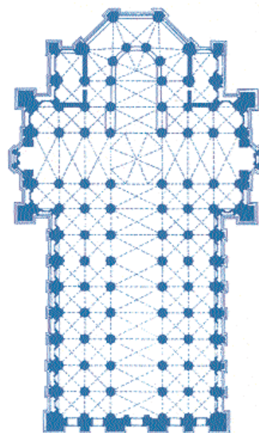
Plan de la Catedral de Milán.
